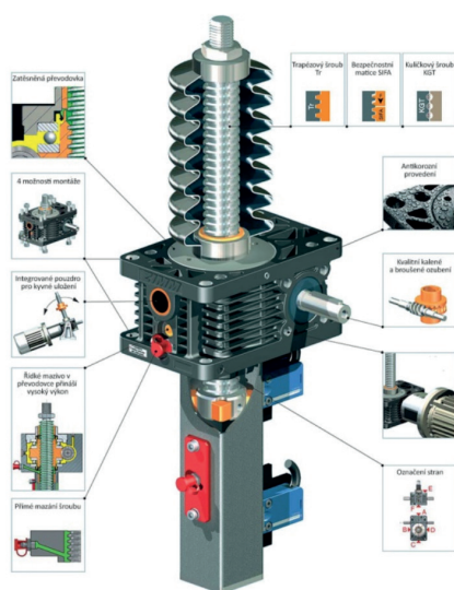
Základní prvky zdvižných převodovek ZIMM série Z
