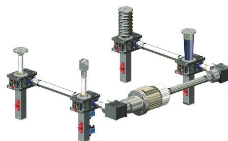
Sestava zdvižných převodovek s ukázkou variability zakončení šroubu
