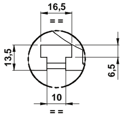
DETTAGLIO / DETAIL Z 1:1
